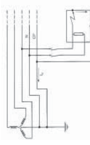
Figura 3. Esquema TN-S.
